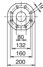
Flanges EN 1092-2 PN 25 - 40
