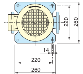
Flanges EN 1092-2 PN 25 - 40
